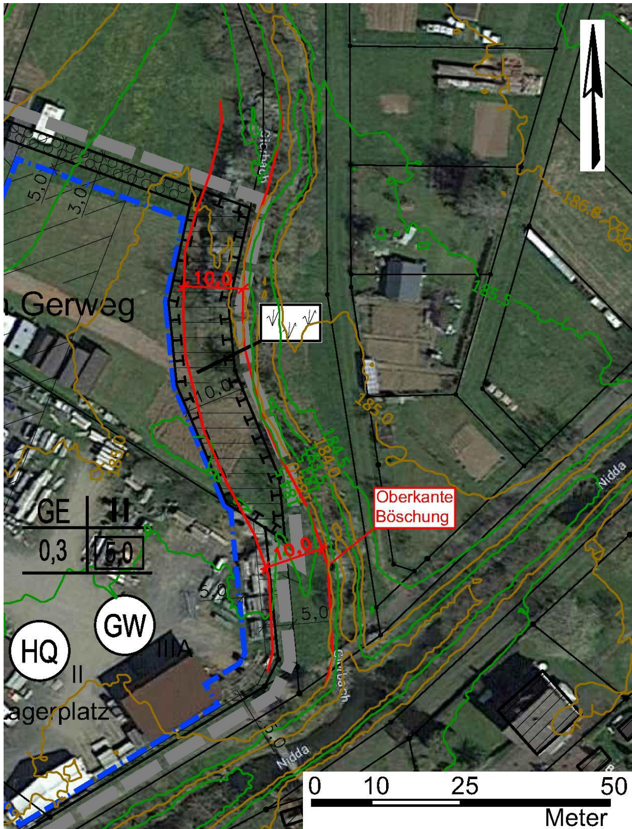
Abbildung 4: Luftbild mit Höhenlinien und eingetragenen 10 m breiten Gewässerrandstreifen (rot dargestellt), überlagert mit den zeichnerischen Festsetzungen des Bebauungsplanes
